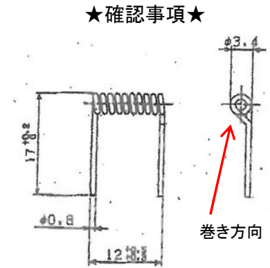
プラズマテック用ストレート GA-001 3.4φ 7.5ターン 幅12.0±0.2 長さ17.0
